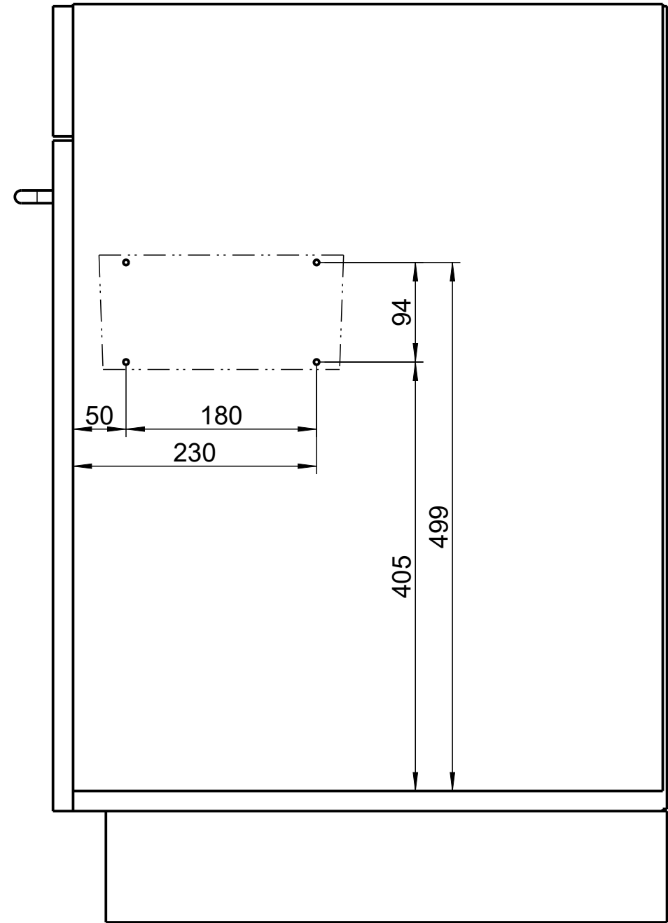
Bohrbilder: Front / Kastenboden / Seitenwand L+R
